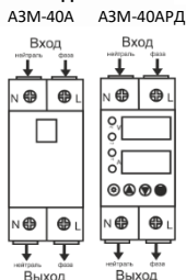
Рис.2 Схема подключения.
