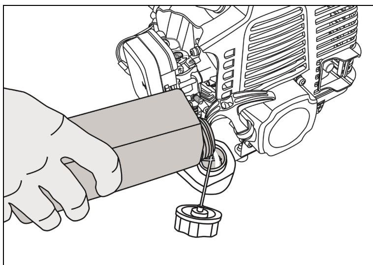
Рис. 15. Заливка топлива
