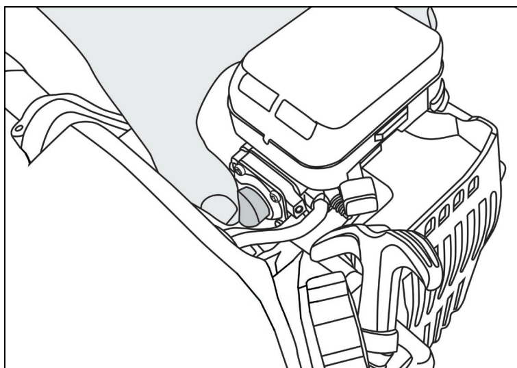
Рис. 19. Подкачка топлива в карбюратор
