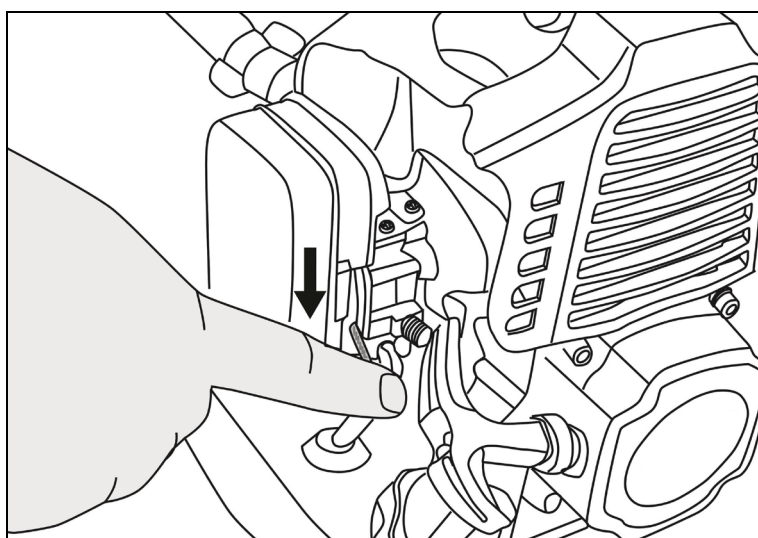
Рис. 23. Открытие воздушной заслонки
