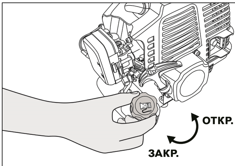
Рис. 14. Откручивание крышки топливного крана
