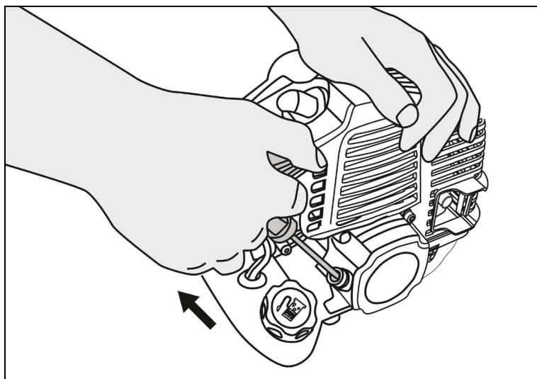
Рис. 22. Запуск двигателя
