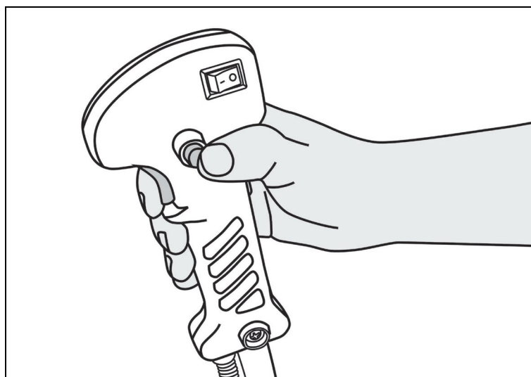
Рис. 27. Фиксация курка газа
